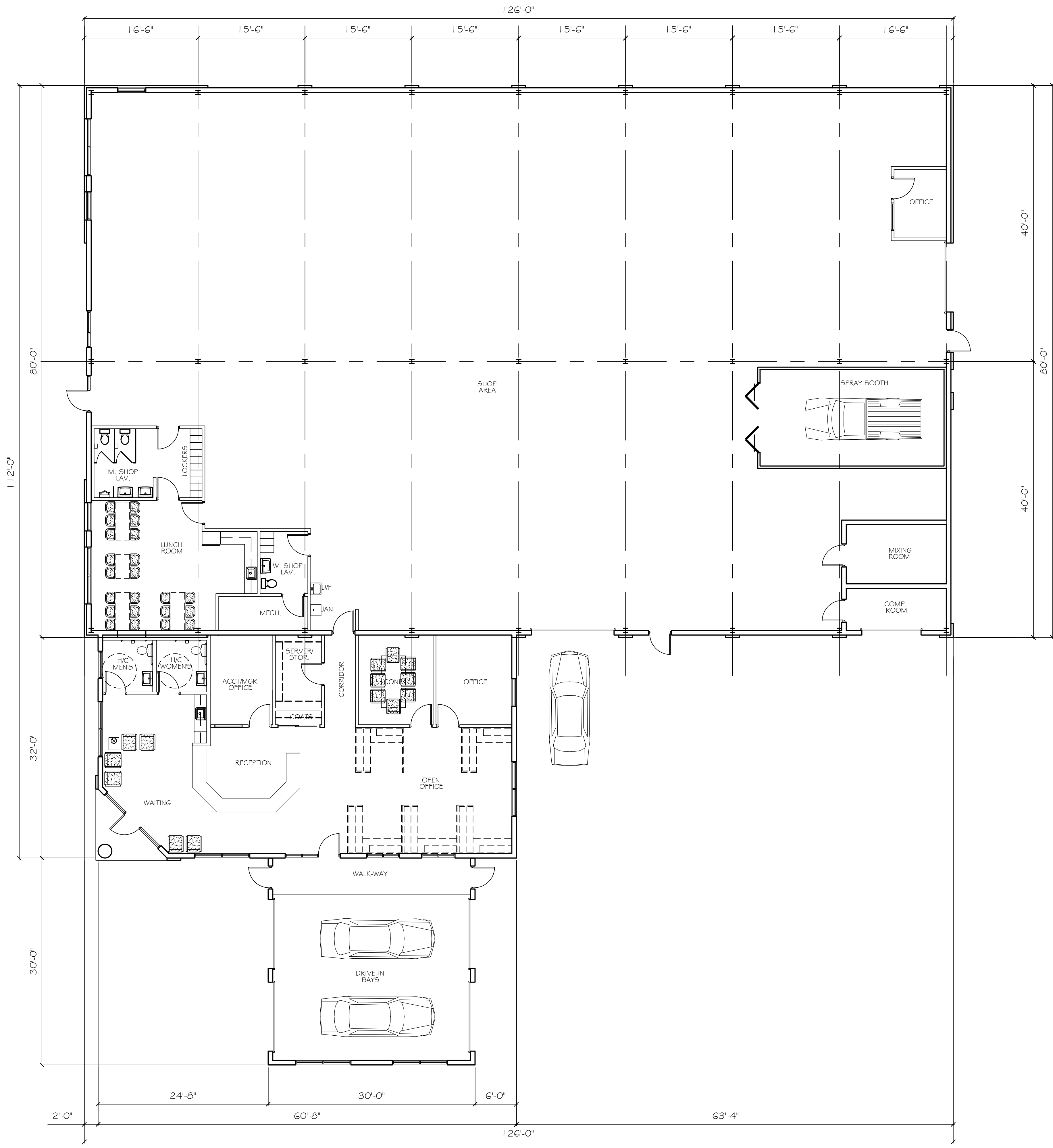
1 FIRST FLOOR PLAN A-1 SCALE: 1/8" = 1'-0"
